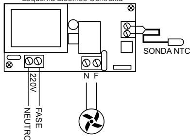
Esquema Electrico Centralita
